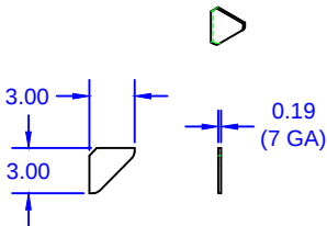
ITEM # 4 (201-52 GUSSET)
